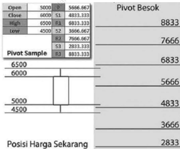
Gambar 3.2 Ilustrasi Pivot
