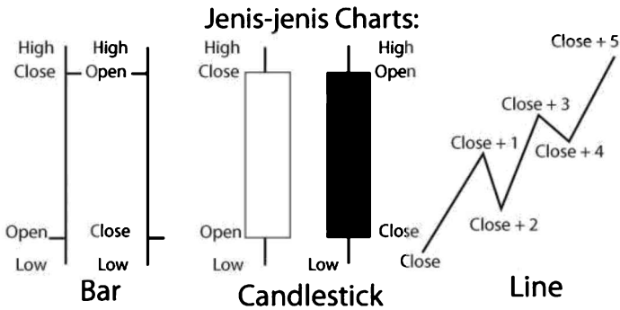
Gambar 2.1 Jenis-Jenis Chart
