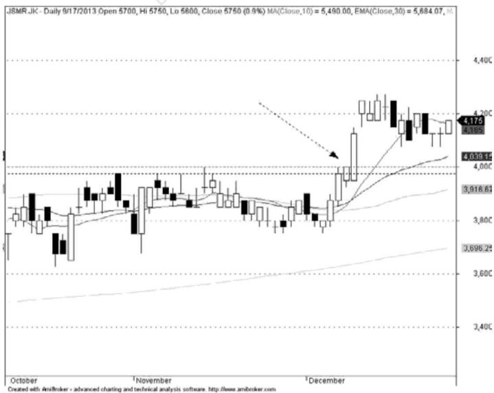
Gambar 8. JSMR Breakout
